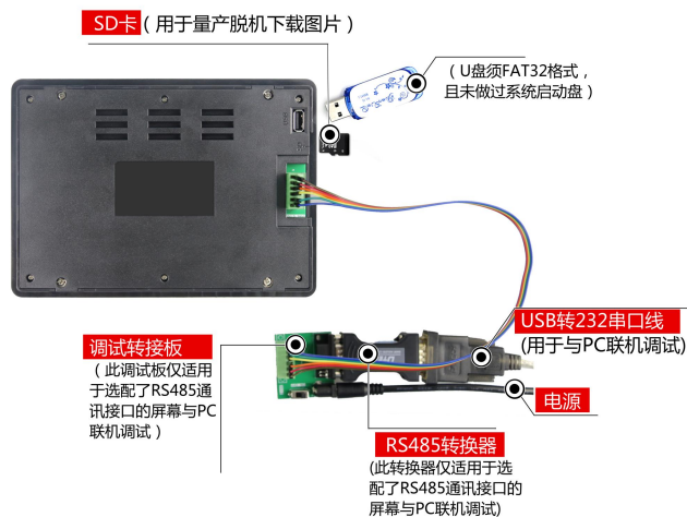
图 1-4 RS485 调试图
