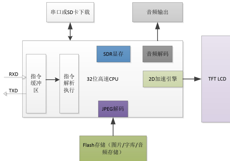
图 12-1 HMI 硬件结构参考图
