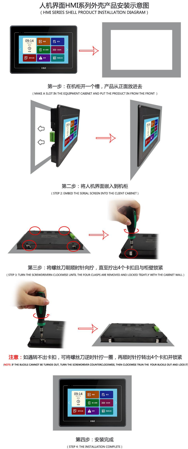
图 2-1 安装示意图
