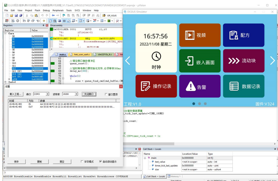
图 13-3Keil 开发环境与虚拟 HMI 绑定调试
