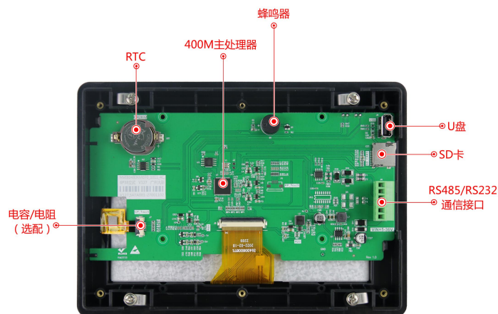
图 1-3 硬件配置图
