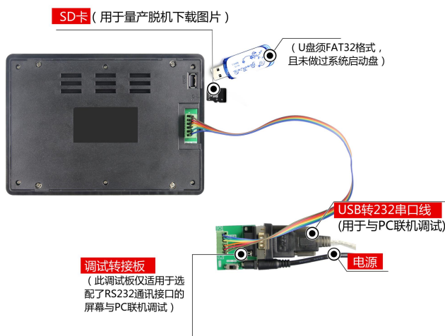
图 1-5 RS232 调试图
