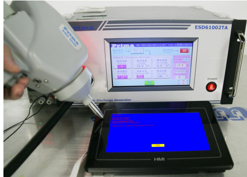
图 7-2 ESD 测试图
