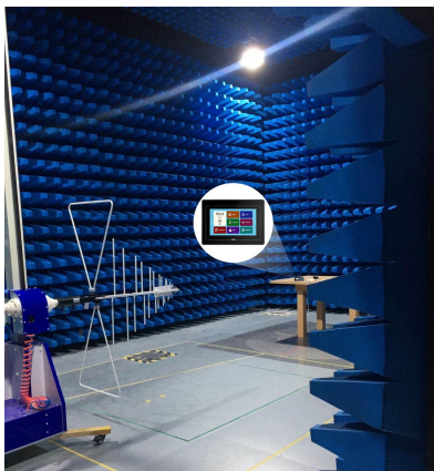
图 7-5 辐射测试图
